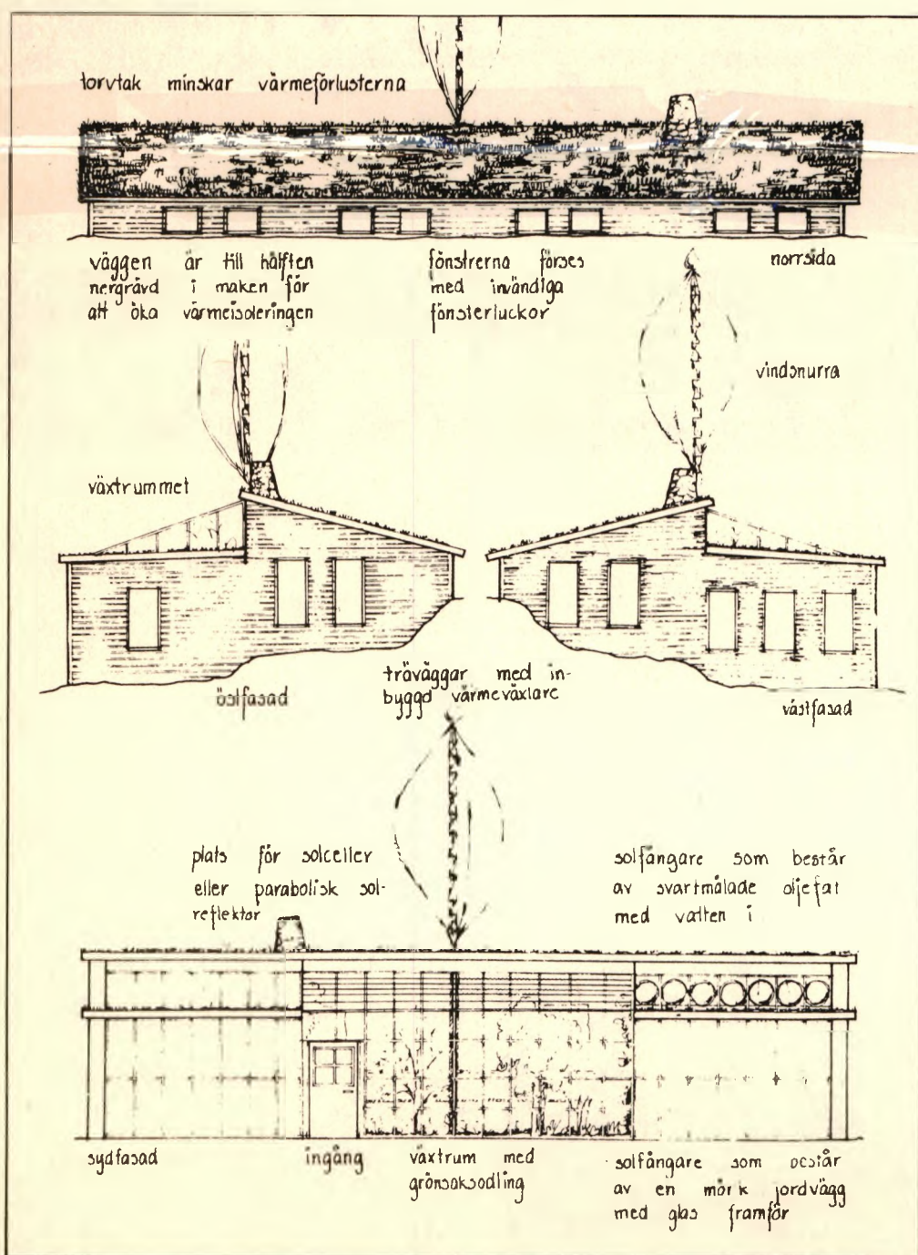
Ekologiskt hus, utarbetat i ett examensarbete av Marita Lorentzon och Egil Öfverholm.
